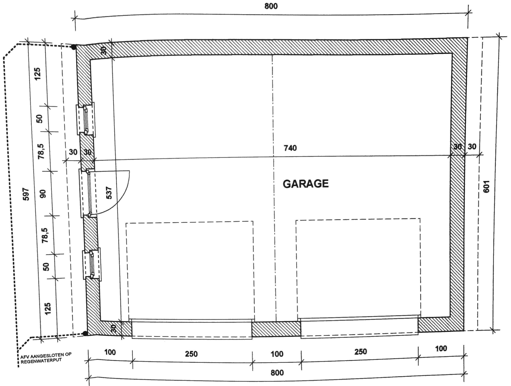
GRONDPLAN 1/50 (nieuwe toestand)
